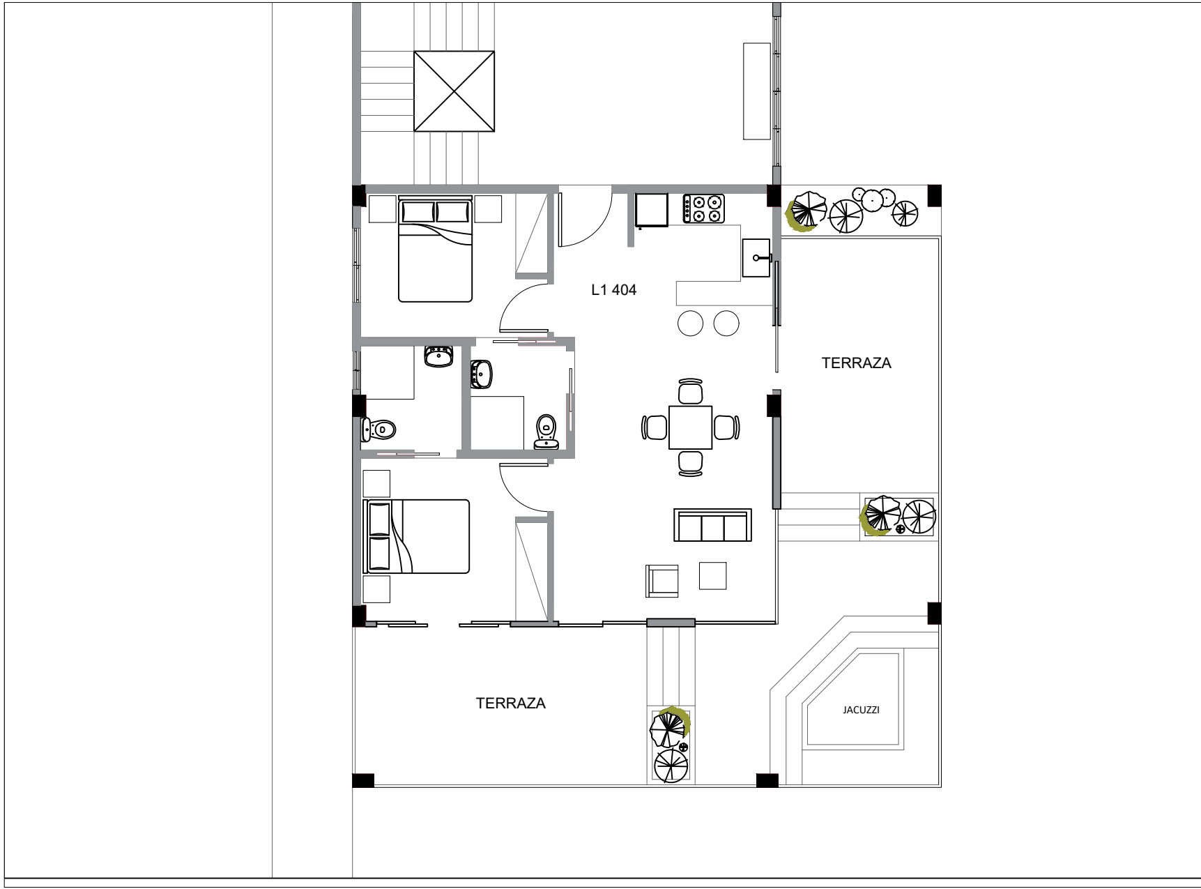
PLANO APTO L1 404 MT2: 120.90
